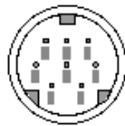
Mini DIN-8 Connector
